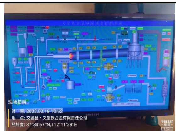
8#回转窑 PLC 控制系统
