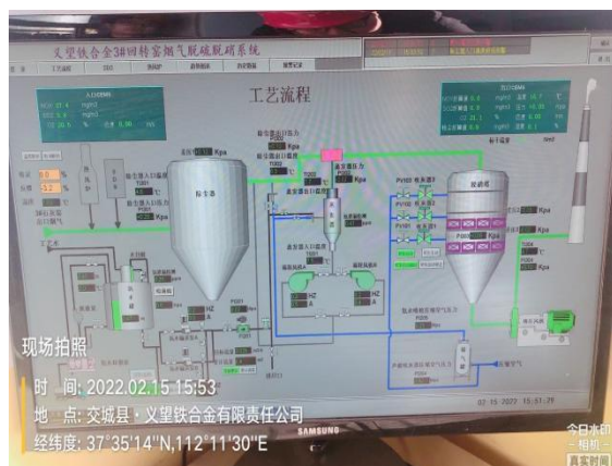
3#石灰石回转窑脱硫脱硝系统 PLC 控制系统及控制柜
