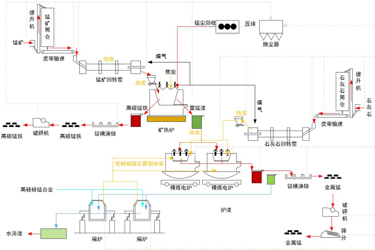
图 2-4 二、三、四分厂工艺流程及排污节点示意图
