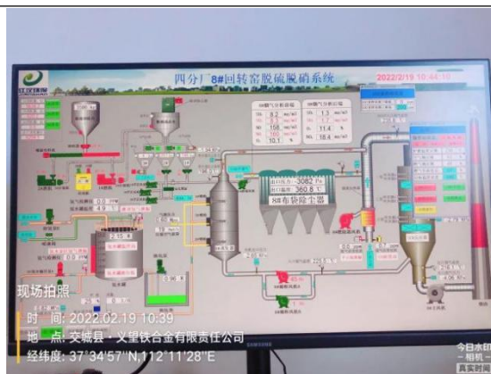
8#回转窑脱硫脱硝 PLC 控制系统
