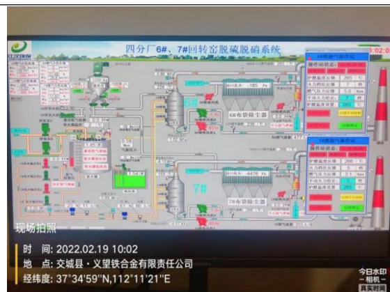
6#、7#回转窑脱硫脱硝 PLC 控制系统
