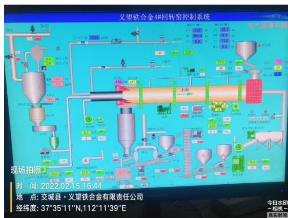
4#锰矿烘干回转窑 PLC 控制系统
