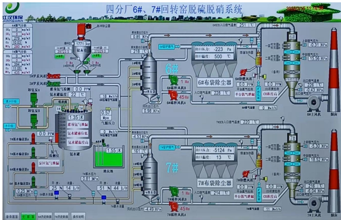
6#锰矿烘干回转窑、7#石灰石回转窑烟气脱硫脱硝系统
