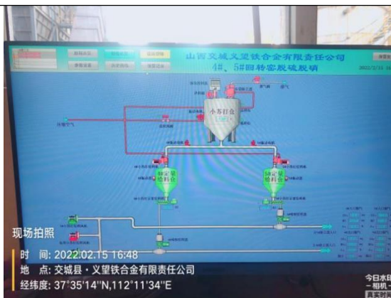
4#、5#回转窑脱硫脱硝系统 PLC 控制系统
