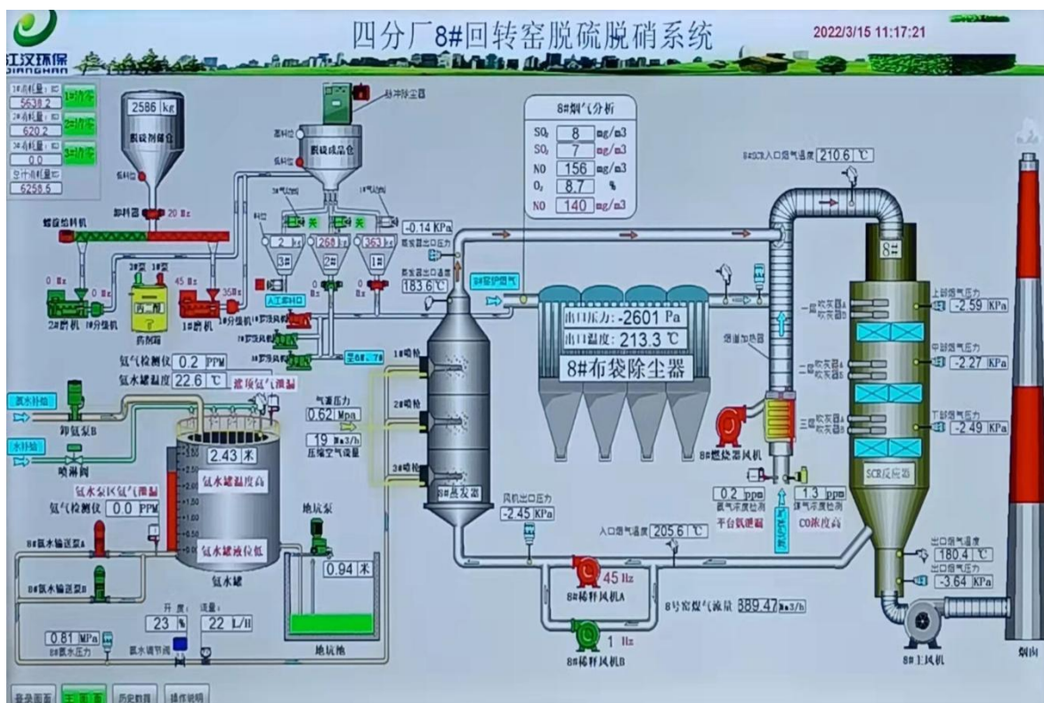
8#回转窑烟气脱硫脱硝系统
