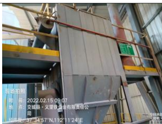
6#、7#回转窑配套脱硫剂料仓及其除尘器
