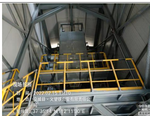
3#回转窑脱硫剂料仓及其除尘器
